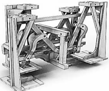
Стопоходящая конструкция Пафнутия Чебышёва, 1878 г.
