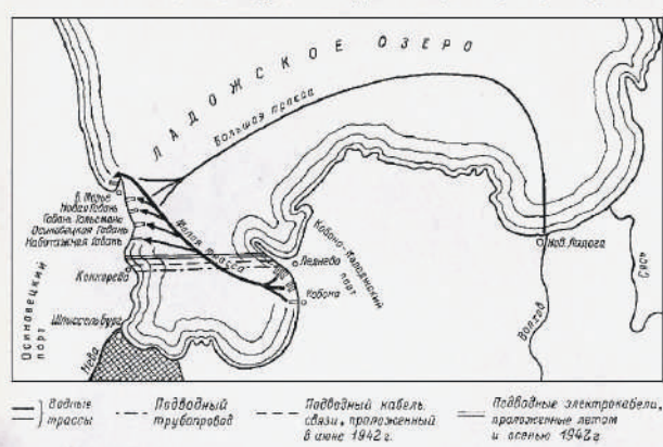
Трубопровод по дну Ладожского озера был построен менее чем за полтора месяца под шквальными обстрелами фашистов. Он стал примером командной работы, которую вели в строгой секретности. Чтобы враг оставался в неведении, освещение не включали и ночью.
