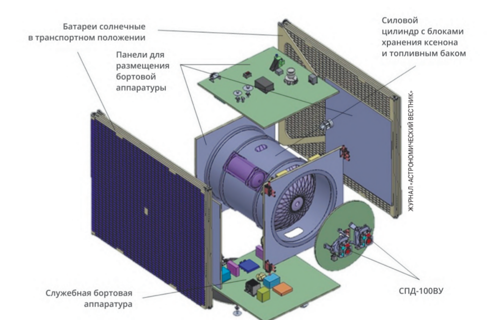
Космический аппарат с электроракетным двигателем.
