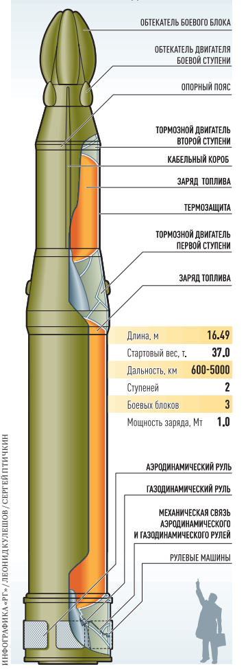
РАКЕТНЫЙ КОМПЛЕКС СРЕДНЕЙ ДАЛЬНОСТИ РСД-10 «ПИОНЕР» (КОД НАТО SS-20 SABER)
